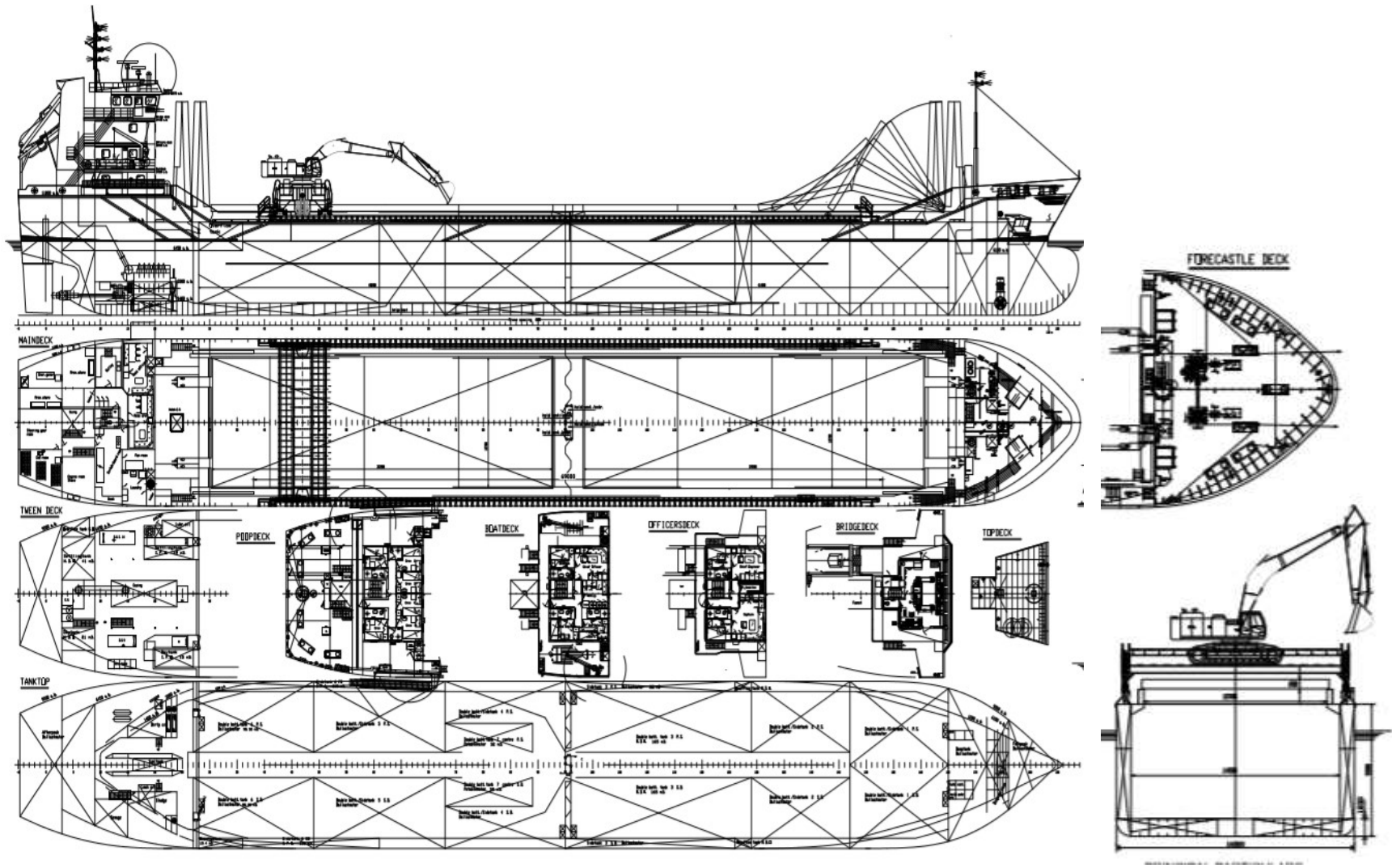
MV 'AASTIND'
